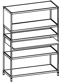
SEC COM010 cm 45x103,4 - h cm 139
